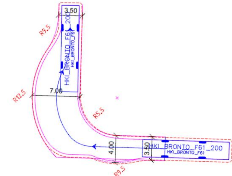
Kuva 1. Nostolavayksikön ajouramalli.
