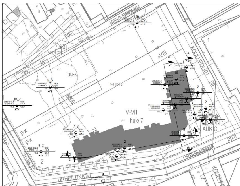
Kuva 1. Ote pohjatutkimuskartasta (Insinööritoimisto Lepistö oy 16.11.2025).
